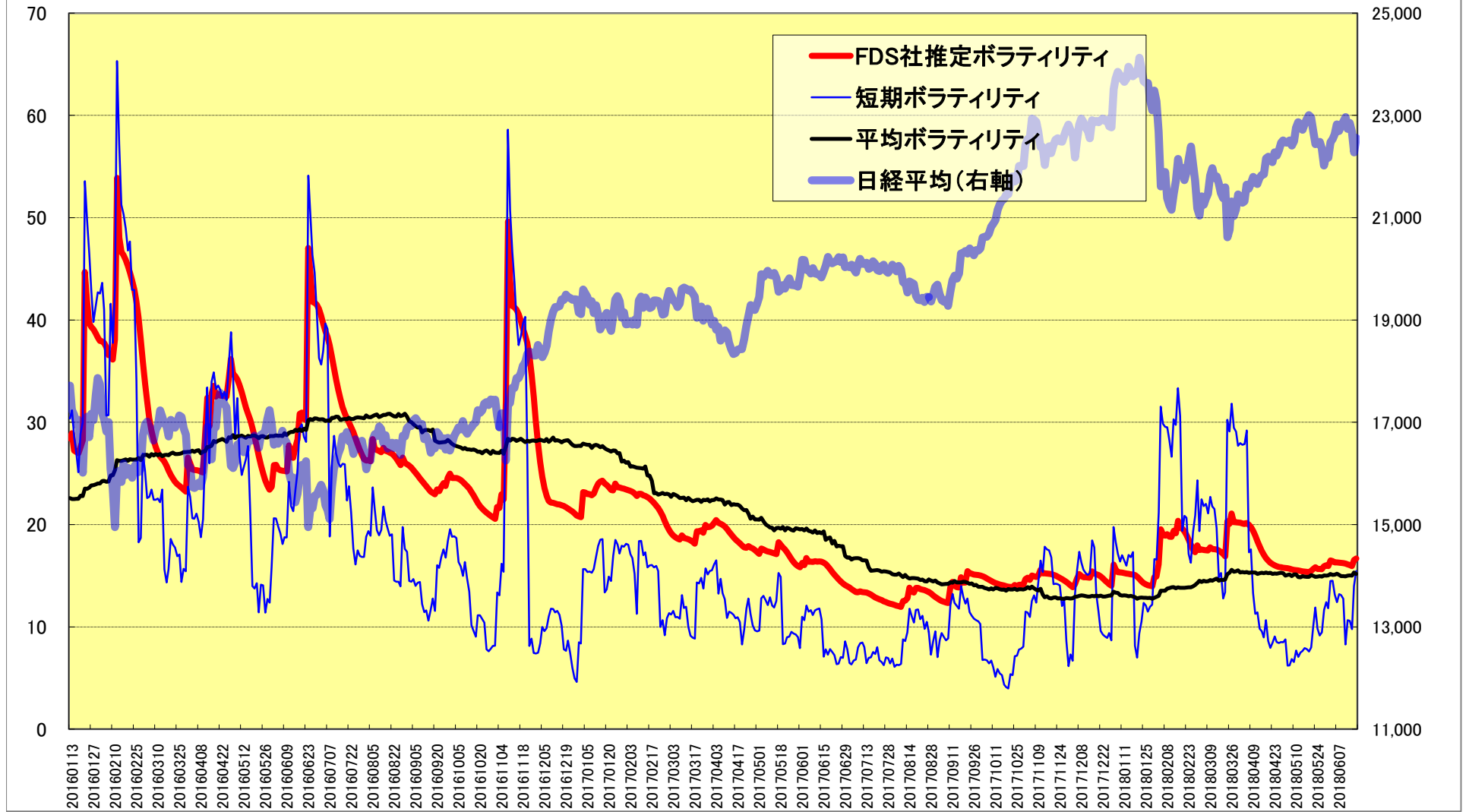
日経平均 FDS社推定ボラティリティ [%/year/ \sigma ] 20160113 ~ 20180620
